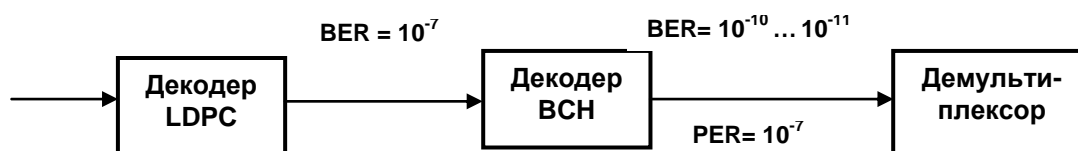
Рис. К.1 – Соотношение битовых и пакетных ошибок в условиях квазибезошибочного приема
