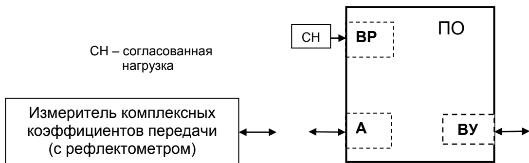
Рисунок 7.7 – Структурная схема для определения затухания несогласованности входа (выхода) приемного оборудования
