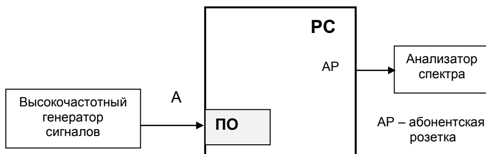
Рисунок 7.1 – Структурная схема для определения неравномерности АЧХ распределительной сети
