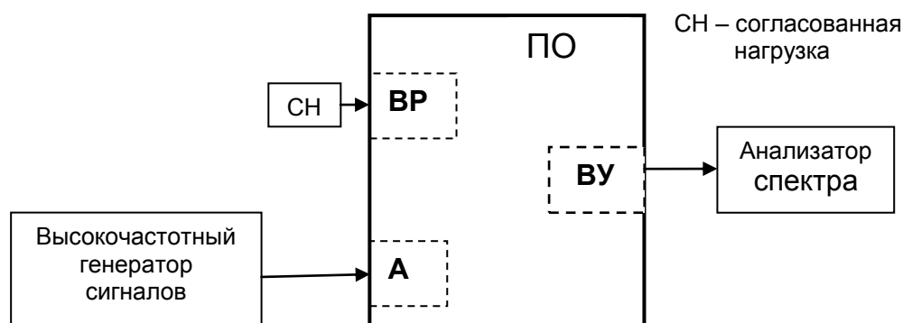
Рисунок 7.5 – Структурная схема для определения диапазона регулировки уровня напряжения радиосигнала на выходе приемного оборудования
