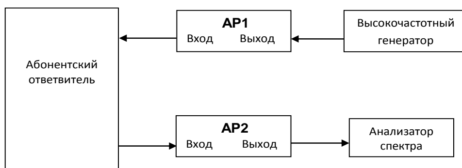
Рисунок 7.3 – Структурная схема для определения переходного затухания между выходами абонентских розеток
