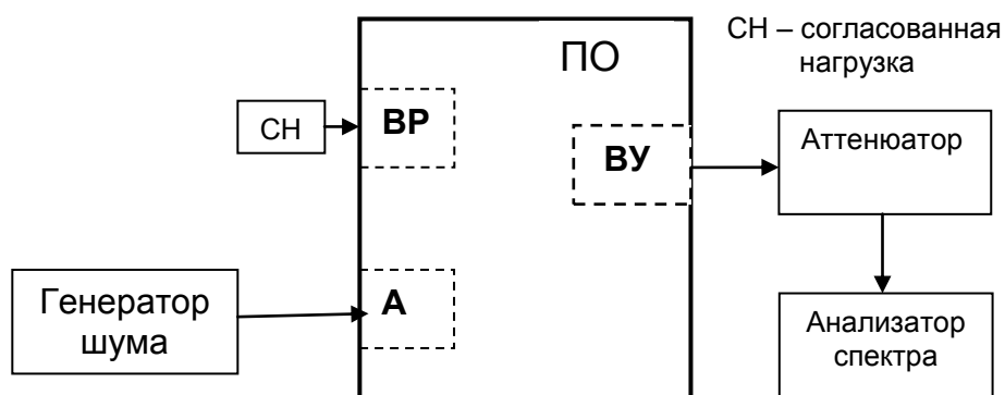
Рисунок 7.4 – Структурная схема для определения коэффициента шума приемного оборудования
