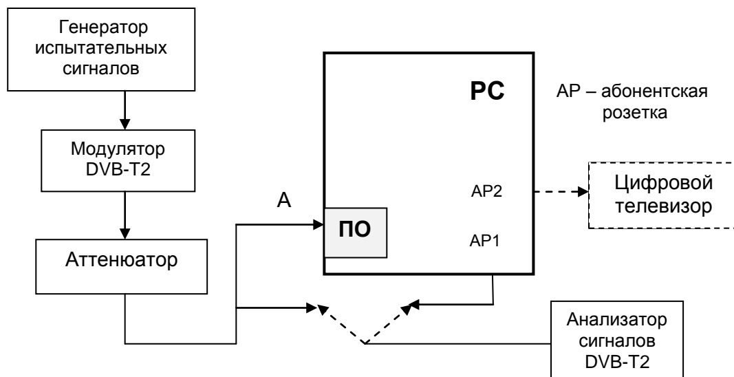
Рисунок 7.2 – Структурная схема для определения отношения радиосигнала к шуму, коэффициента битовых ошибок и субъективной оценки качества изображения и звукового сопровождения на выходе распределительной сети
